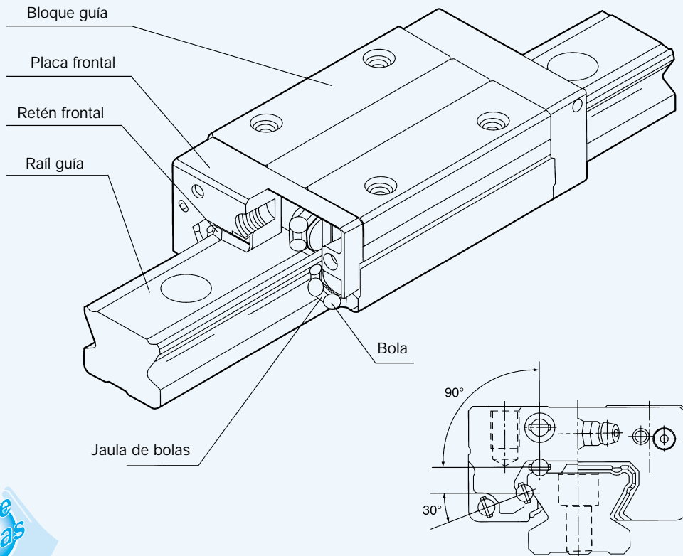
Figura 1 ■ Corte transversal del tipo SSR-XW.
